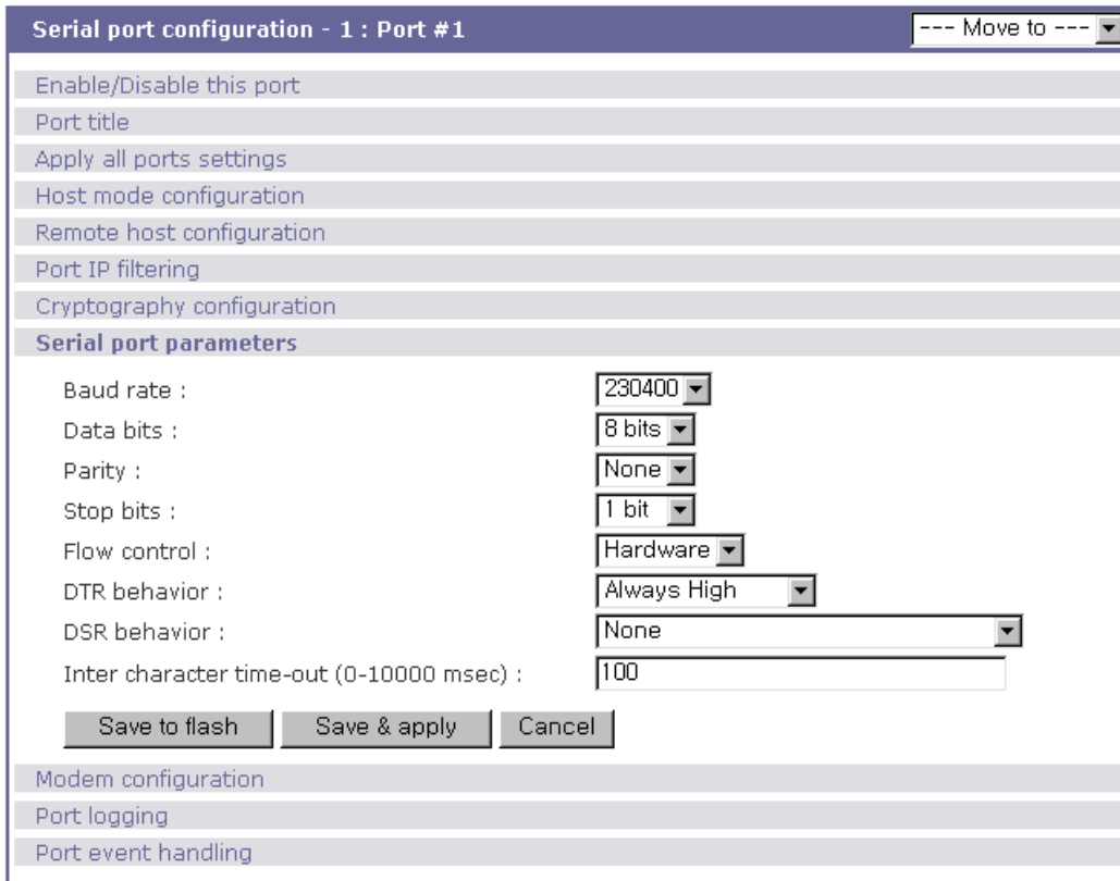
그림 4-15 UART 설정
