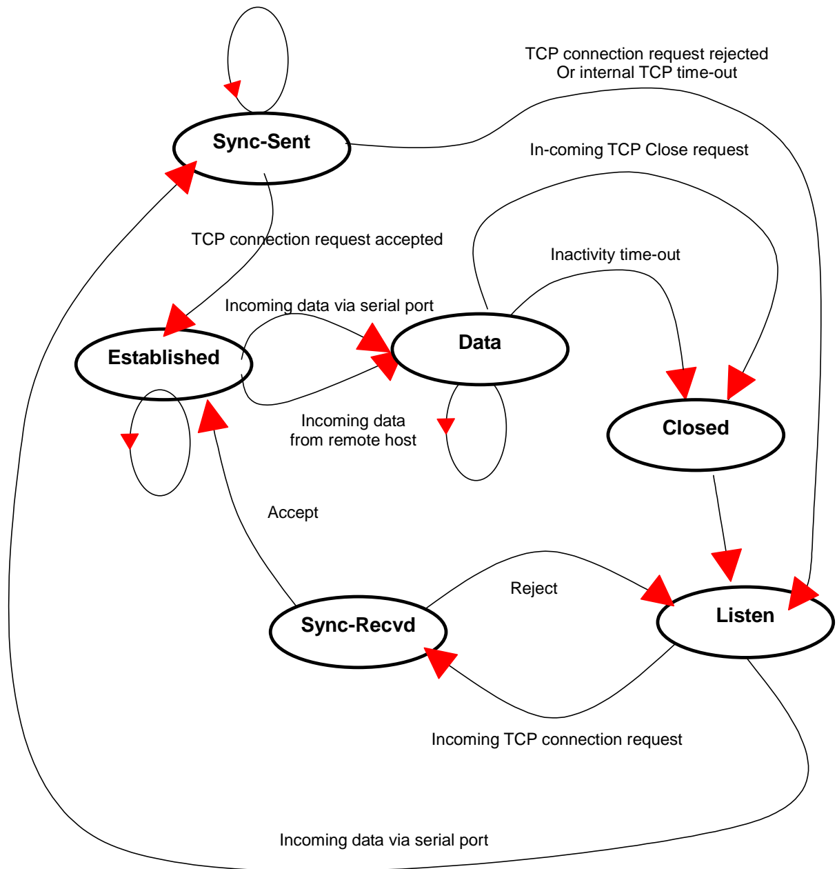
그림 4-6 TCP모드의 상태전이도
