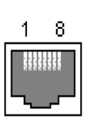
그림 A-1 RJ45 커넥터의 핀 배치
