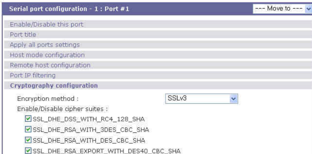
그림 A-12 암호기법 설정( Cryptography configuration)
