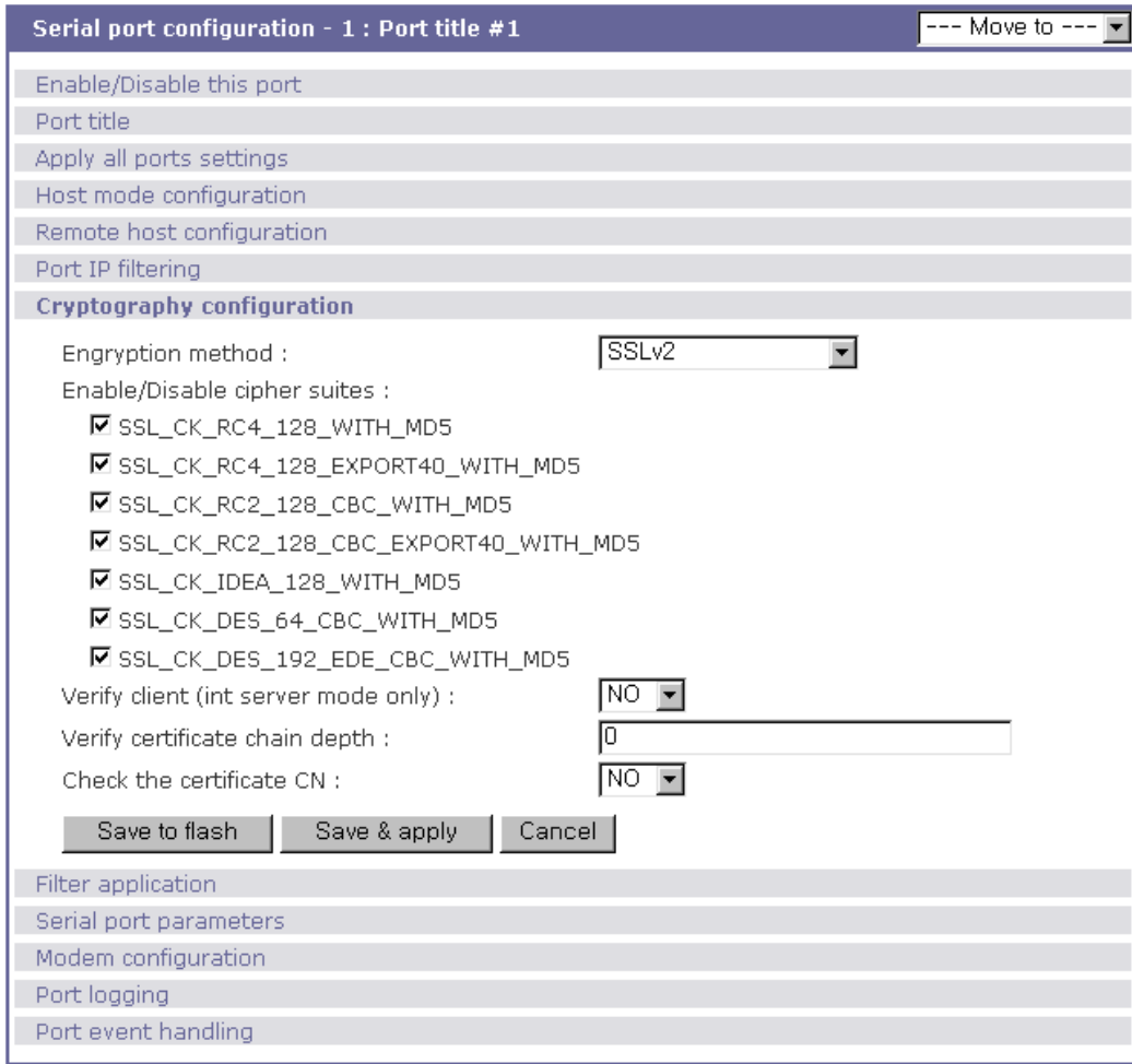
그림 4-11 암호화 구성
