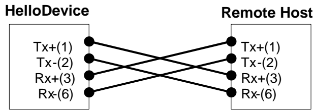
그림 A-2 Ethernet direct connection using crossover Ethernet cable
