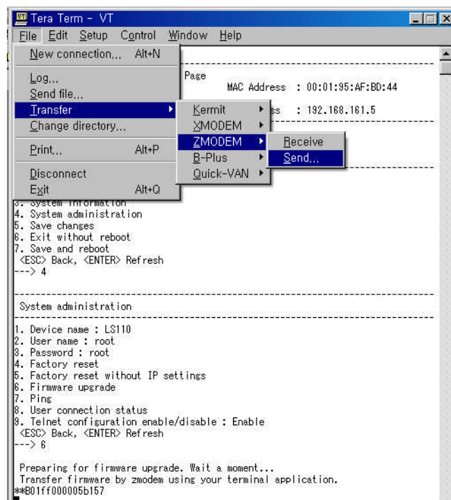
그림 6-8 ZMODEM 실행화면
