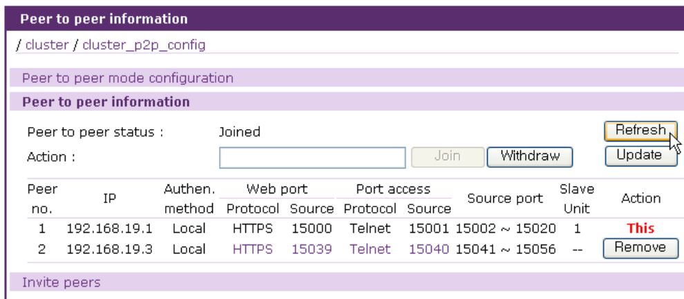
그림 5-17 Clustering Peer-to-peer – Join 완료 후 Join 대상 peer의 화면
