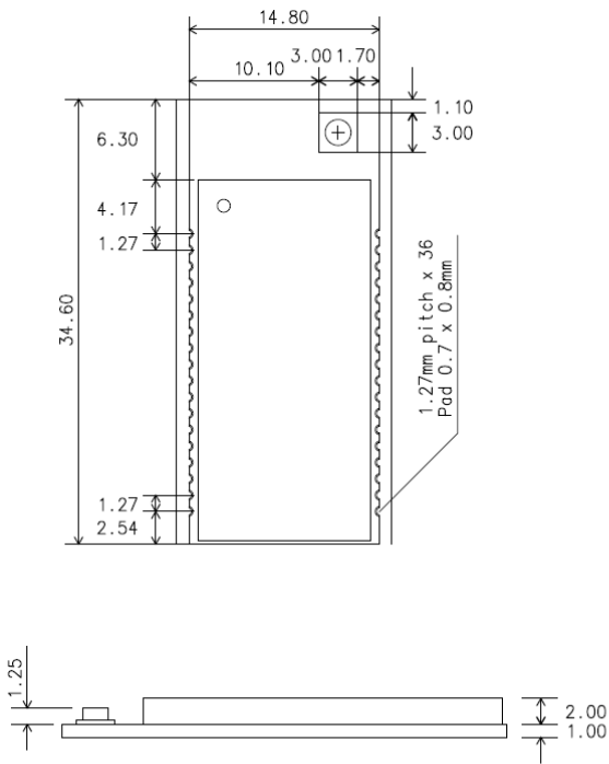
그림 1-3 BCD110SU 치수
