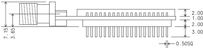
그림 1-7 BCD110DS 치수
