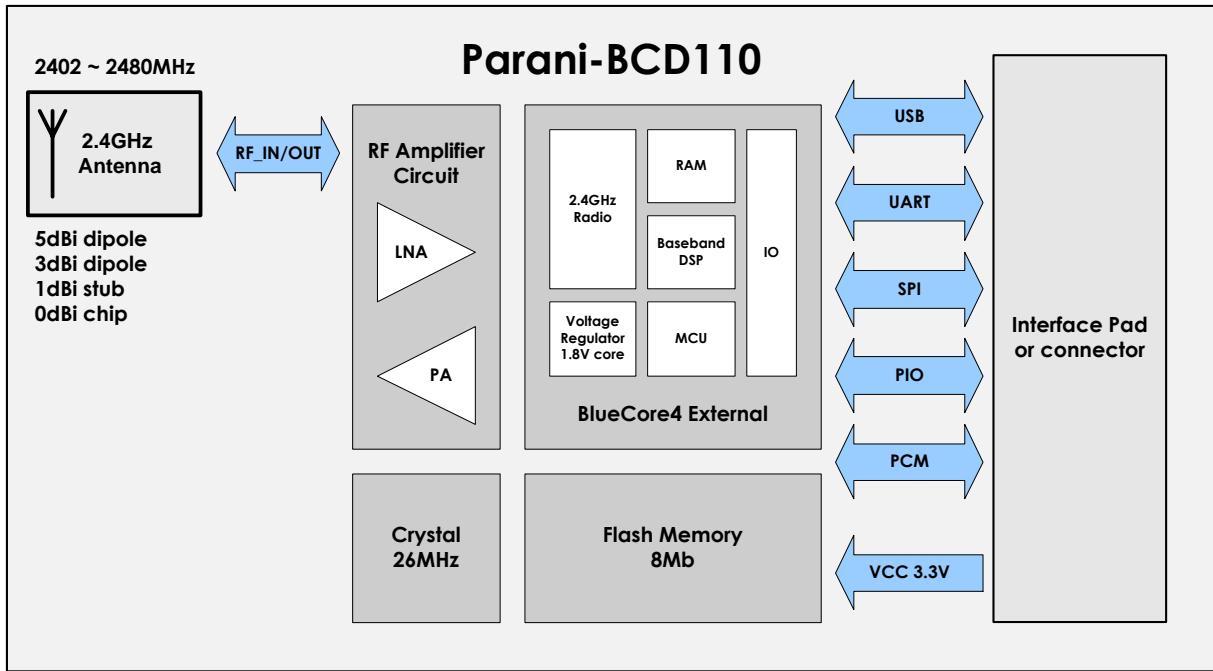
그림 1-1 블록 다이어그램
