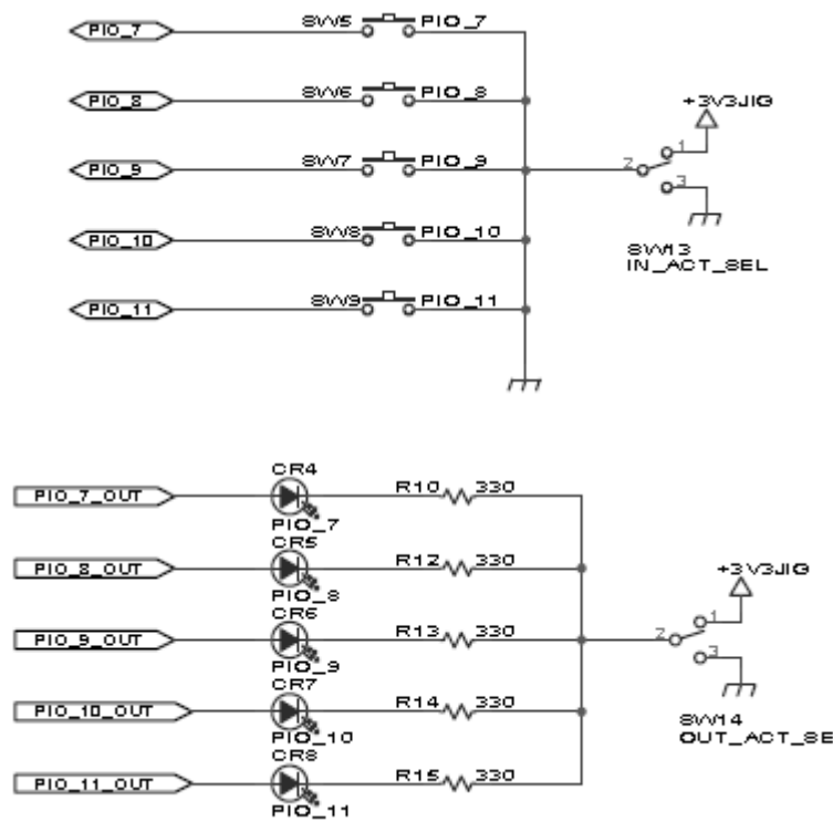
그림 5-6 GPIO 인터페이스
