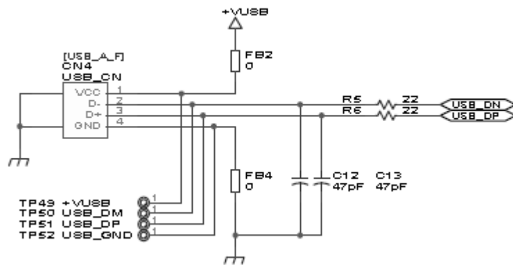
그림 5-7 USB 인터페이스
