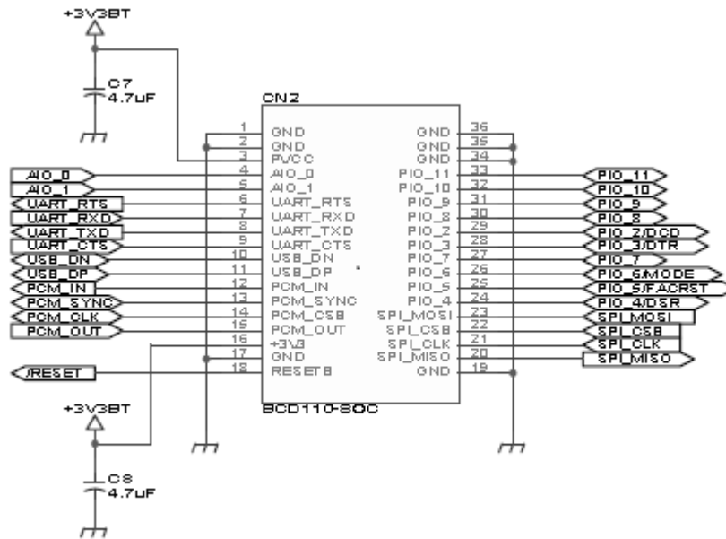
그림 5-1 BT 모듈 인터페이스
