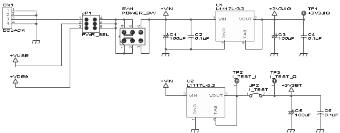
그림 5-2 전원 및 리셋 인터페이스
