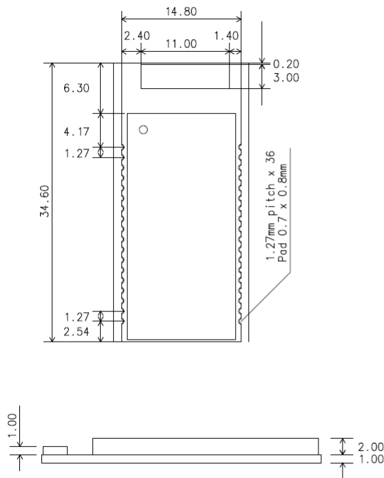
그림 1-3 BCD110SU 치수
