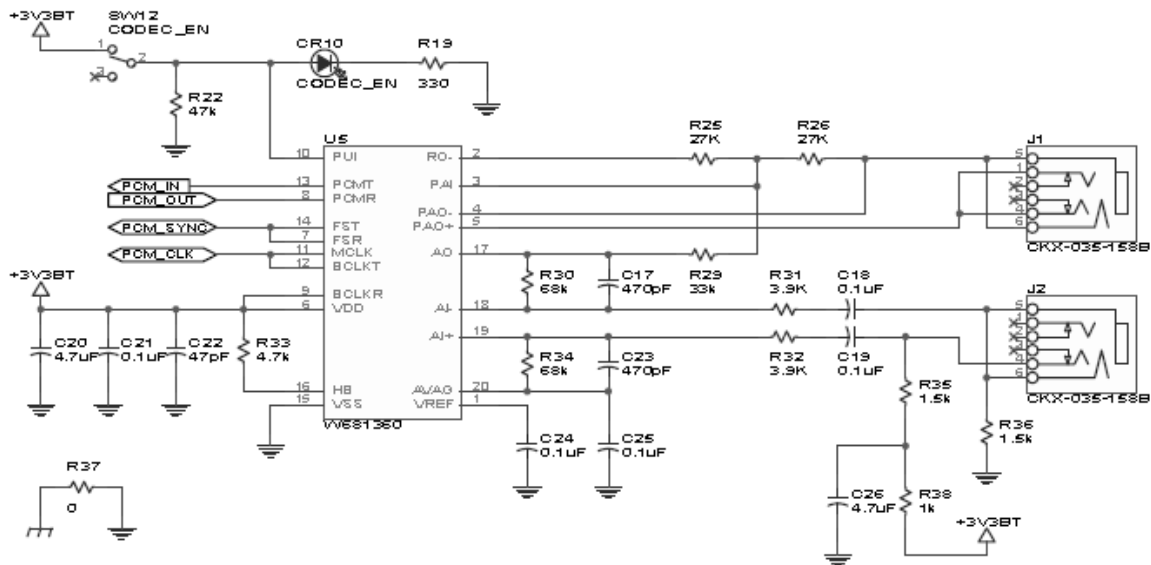
그림 5-9 PCM 인터페이스
