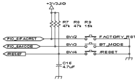
그림 5-5 스위치 인터페이스
